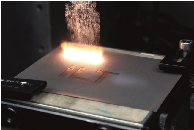
Bild 2: Strukturierung von Elektroden: Abtrag des Aktivmaterials auf einer Kupferfolie. © Fraunhofer ILT, Aachen.
