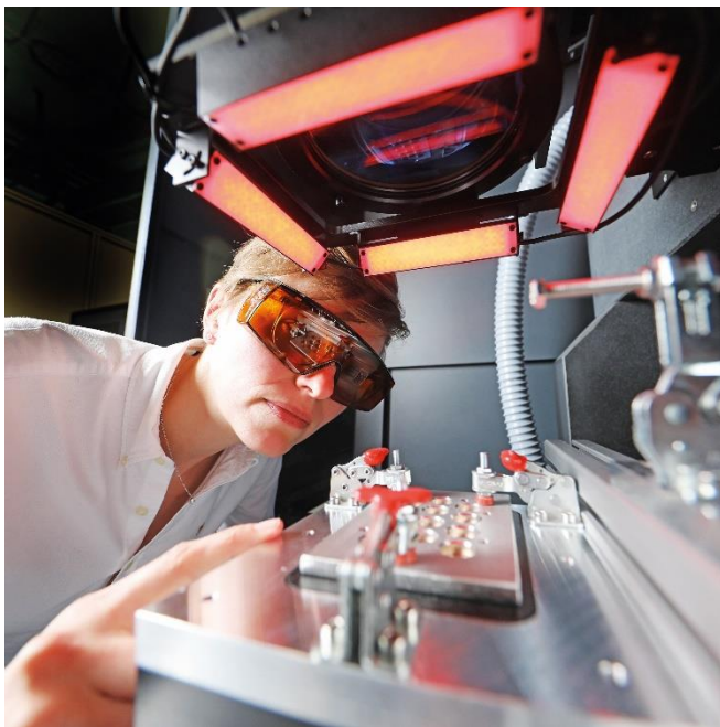
Bild 3: Einrichtung der Laserschweißmaschine für die Herstellung von Batteriemodulen. © Fraunhofer ILT, Aachen / Andreas Steindl.
